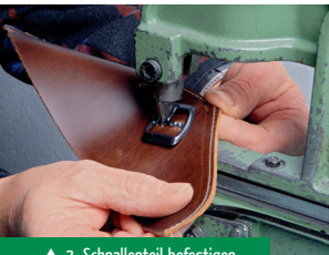
▲ 3. Schnalle Teil befestigen
